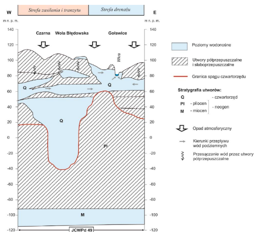
Rysunek 9. Schemat krążenia wód podziemnych JCWPd nr 49
