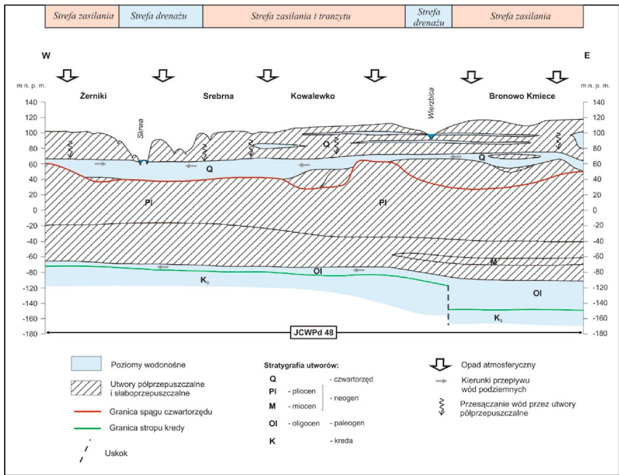
Rysunek 8. Schemat krążenia wód podziemnych JCWPd nr 48 Źródło: PSH
